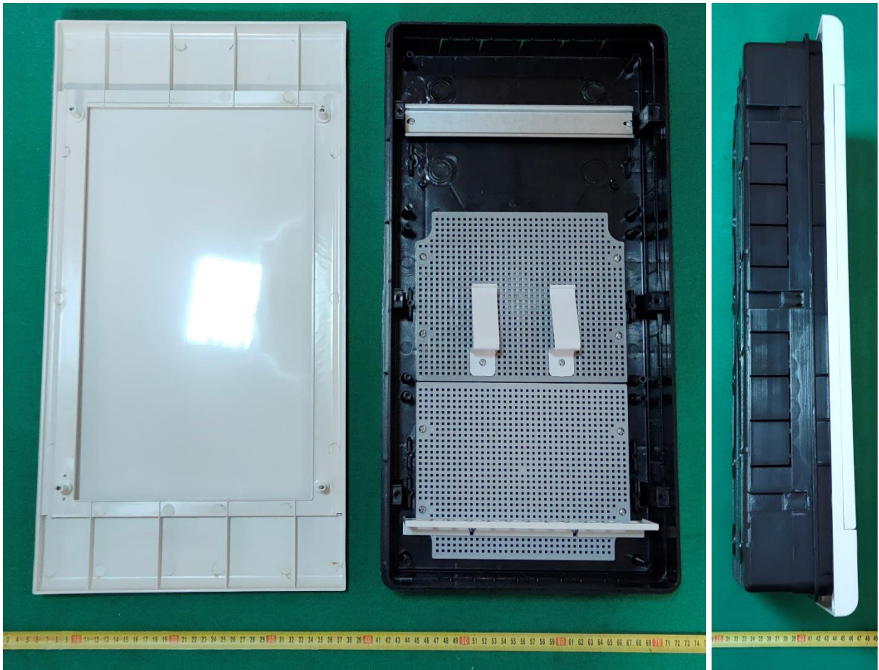
Obudowa typu SRp-36/BM
